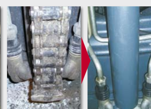
Hydraulik am Hubmast
